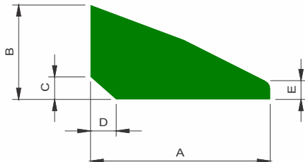
PERFIL TRIANGULAR AÉREO
