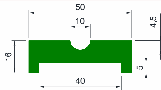
PERFIL AÉREO
