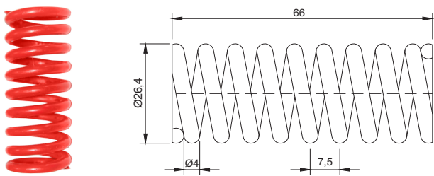
MOLA PARA CAPSULADOR
