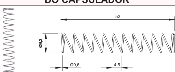
MOLA PARA ARROLHADOR DO CAPSULADOR
