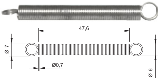
MOLA DO DISTRIBUIDOR DE ROLAS DO CAPSULADOR
