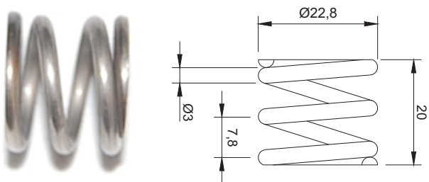
MOLA PARA O CABEÇOTE DO CAPSULADOR
