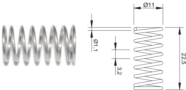
MOLA PARA CAPSULADOR
