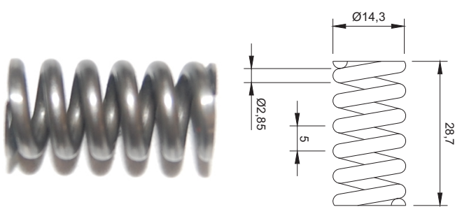
MOLA INTERNA DO CAPSULADOR
